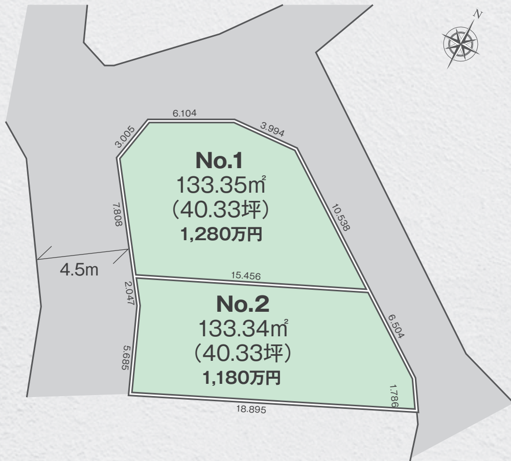
区画図
